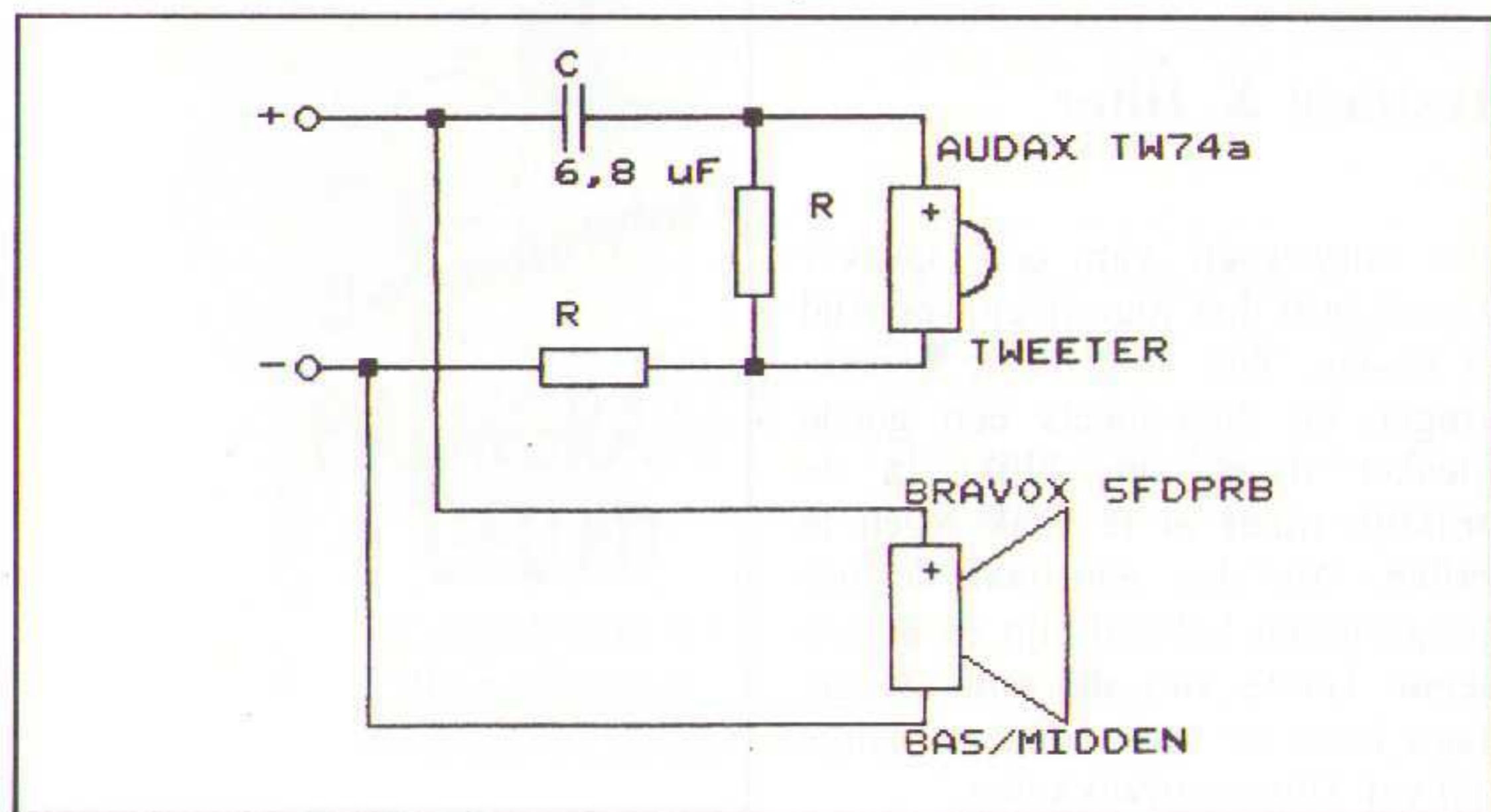
Figuur 1. Het filter van 'Freek'.
